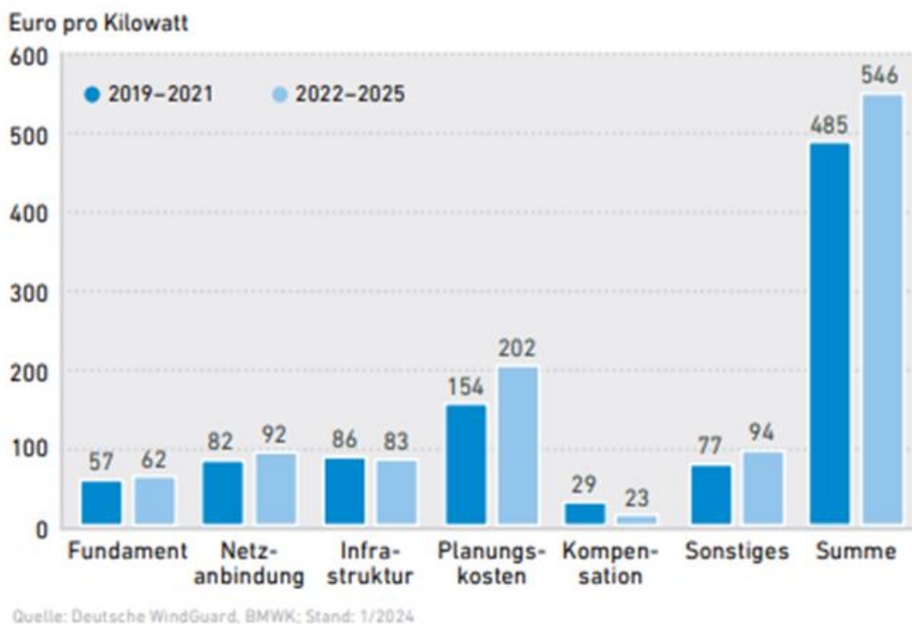
Abbildung 55: Entwicklung von Nebeninvestitionskosten On-Shore Wind Quelle: AEE (2024)
