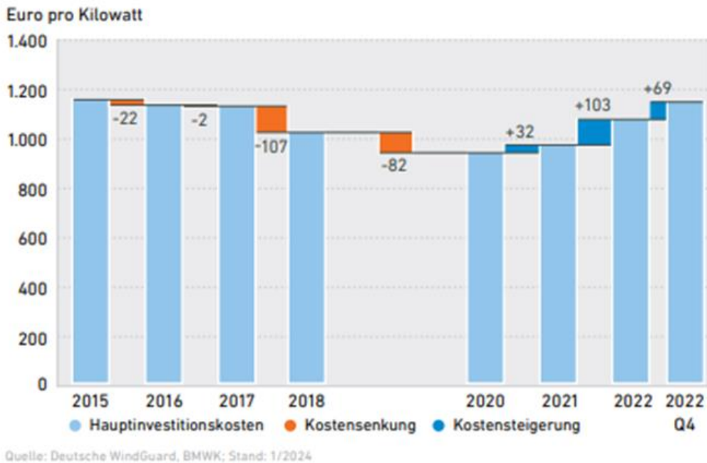
Abbildung 54: Entwicklung von Hauptinvestitionskosten On-Shore Wind Quelle: AEE (2024)
